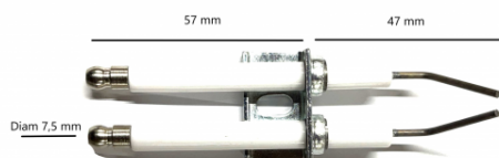
Electrode double pour chaudière NHP Annovi type 6640, 6670, 7950, 7870, 8860, 8870.
